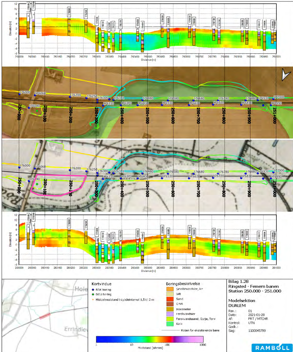
Figur 2-3: Eksempel fra de undersøgelser, som er foretaget langs banen, hvor der både er vist oplysninger fra boringer og fra de geofysiske undersøgelser. Graveområdet er markeret med pink på figuren.
