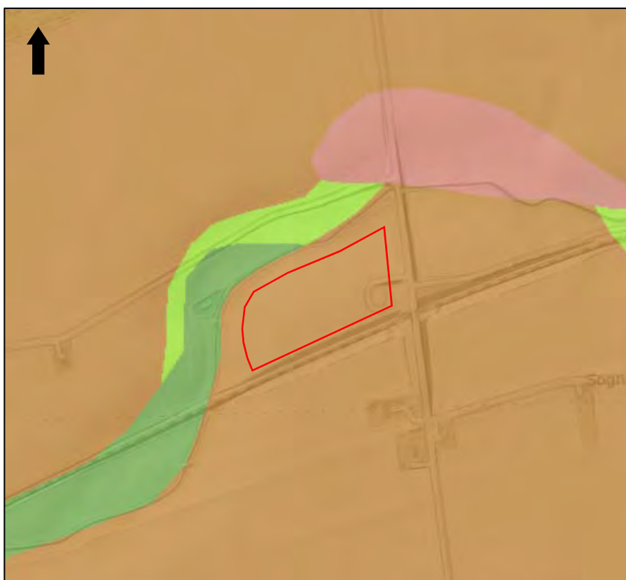
Figur 4. Jordartskort (1:25.000) som viser geologien i den øverste meter af jordoverfladen. Moræneler (brun), smeltevandssand (lyserød) og ferskvandsaflejringer i form af tørv (mørk grøn) og ferskvandssand (lys grøn). Graveområdet er markeret med rødt.
