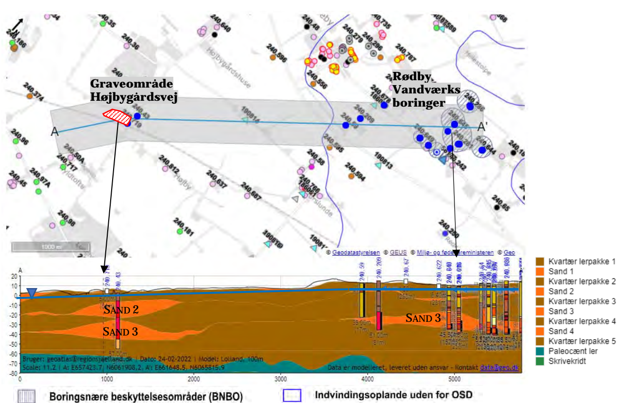
Figur 5. Geologiske profil fra Hylldtofte (til venstre), gennem graveområde Højbygårdsvej og til Rødby Vandværks boringer (til højre). Grundvandsspejlet for det primære magasin (Sand 3) er vist med blå linje i profilet. X-aksen viser afstanden i meter og y-aksen viser dybden i kote m DVR90. Geologisk model: Lolland, 100 m. Kilde: GeoAtlas Live.
