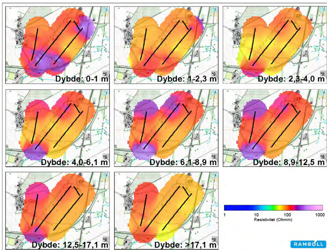
Figur 3.4: Middelmodstandskort for de enkelte modellag i 8-lagstolkningen.
