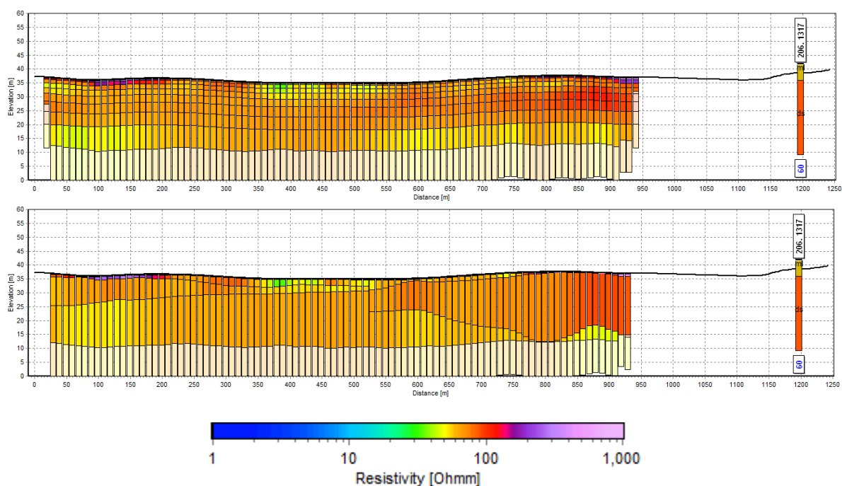
Figur 3.5: Øverst ses placeringen af profil E1, øst for Glim. Dernæst ses hhv. manglagstolkningen, og 3-lags tolkningen af de, langs profilet, indsamlede PACES-data. Boringer er projiceret ind langs profilet med en maksimal afstand af 200 m. Projiceringsafstanden er angivet under boringerne, og indtrængningsdybden (DOI) er markeret med en fadet farveskala. Profilet er præsenteret fra Sydvest mod nordøst.
